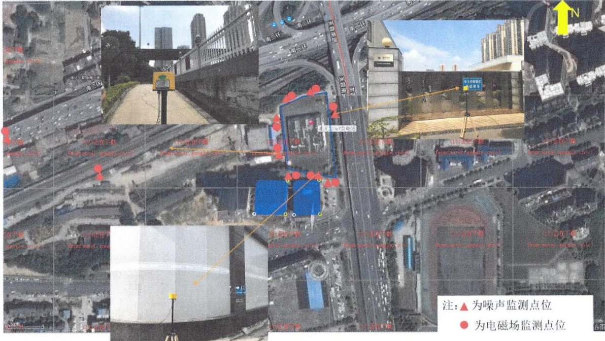
图 8 浦沅 220kV 变电站平面布置及监测点位示意图
