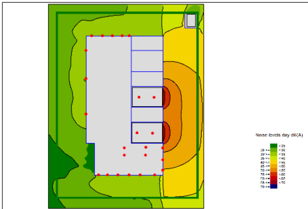
图 7 高丰 220kV 变电站本期规模噪声预测等值线图
