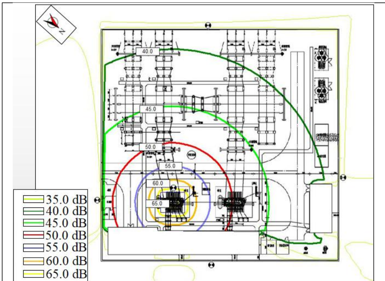
图 7-1 梅溪 110kV 变电站本期规模噪声预测等值线图
