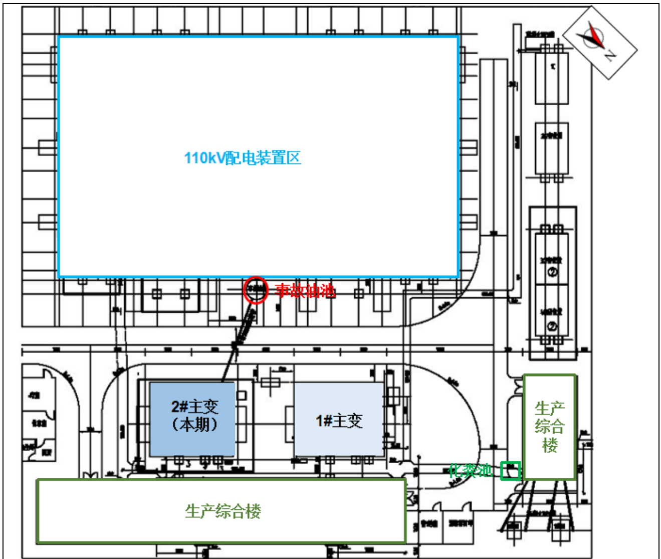
图 1-2 梅溪 110kV 变电站总平面布置图
