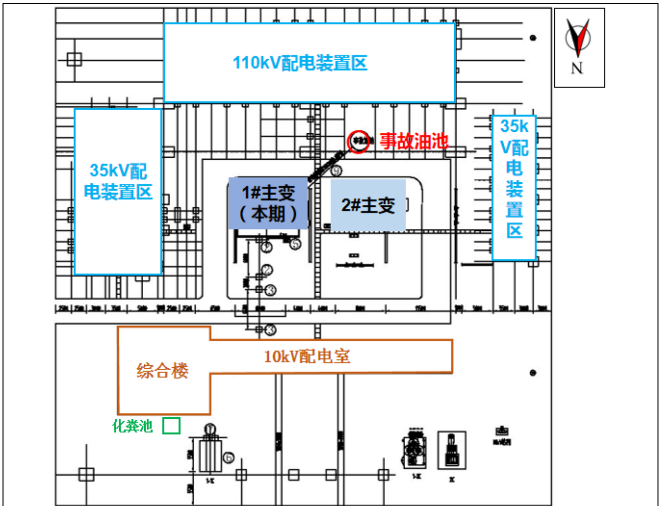
图 1-2 新田 110kV 变电站总平面布置图
