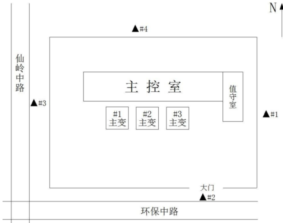
图 4 仙姑岭 110kV 变电站平面布置及监测点位示意图
