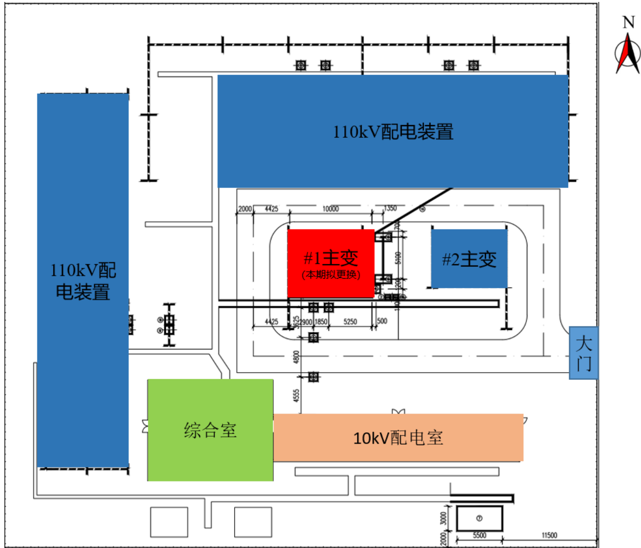
附图2 官山 110kV 变电站总平面布置图
