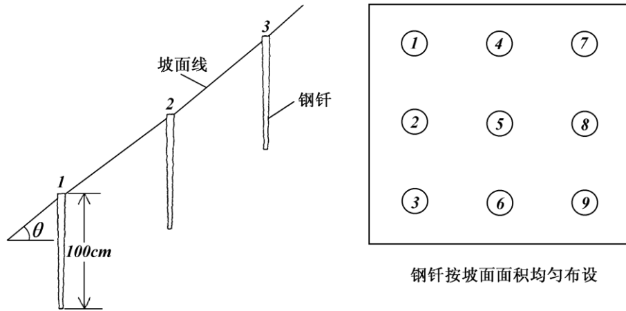
图 3.4-1 简易坡面量测法示意图-测钎法
