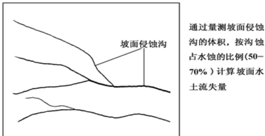
图 3.4-2 简易坡面量测法示意图-侵蚀沟法
