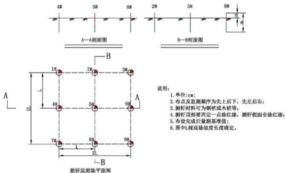
测钎法监测场典型设计图
